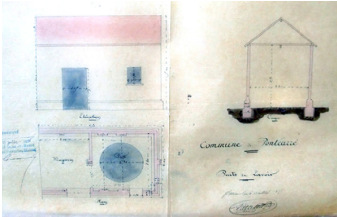
Coupe du lavoir.
